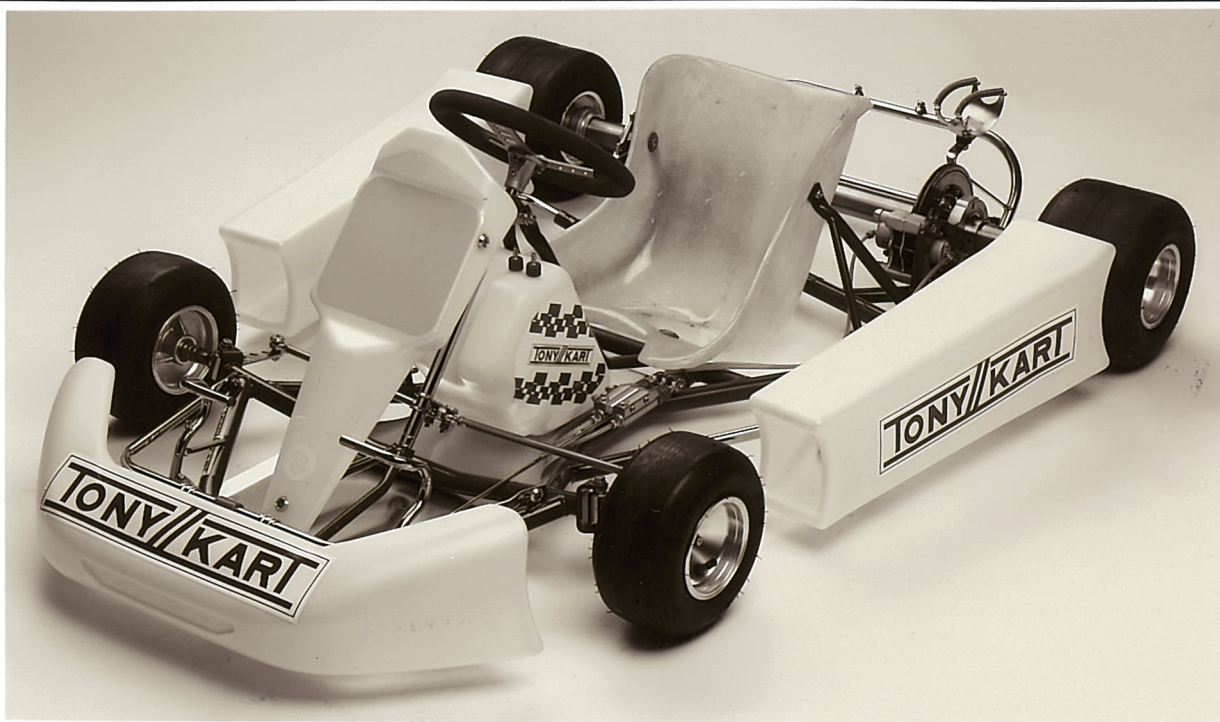
Photo du Kart avec carrosserie et pneumatiques
